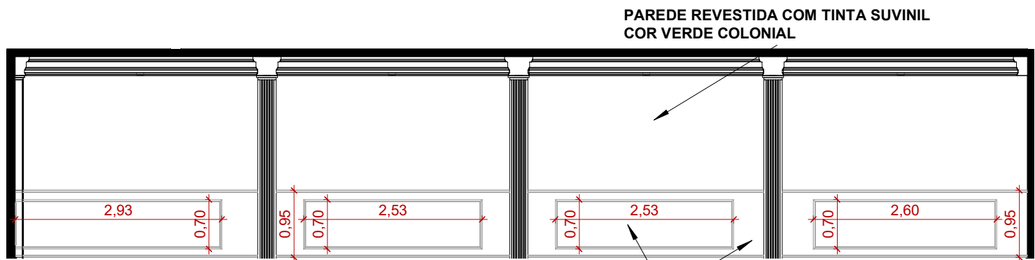
2 BAR - ELEVÇÃO FRONTAL 1 : 75
