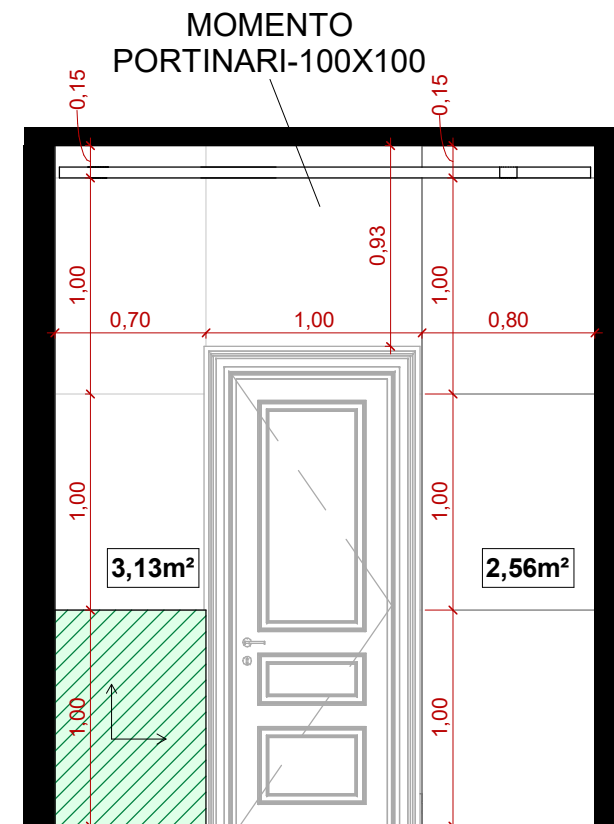
3 WC 03 - ELEVÇÃO POSTERIOR 1 : 35
