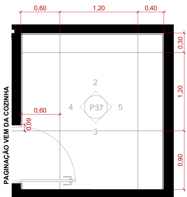
1 DEPÓSITO (COZINHA) - PAGINAÇÃO 1 : 35
