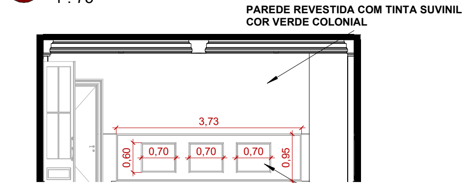
4 BAR - ELEVÇÃO LAT. ESQUERDA 1 : 75
