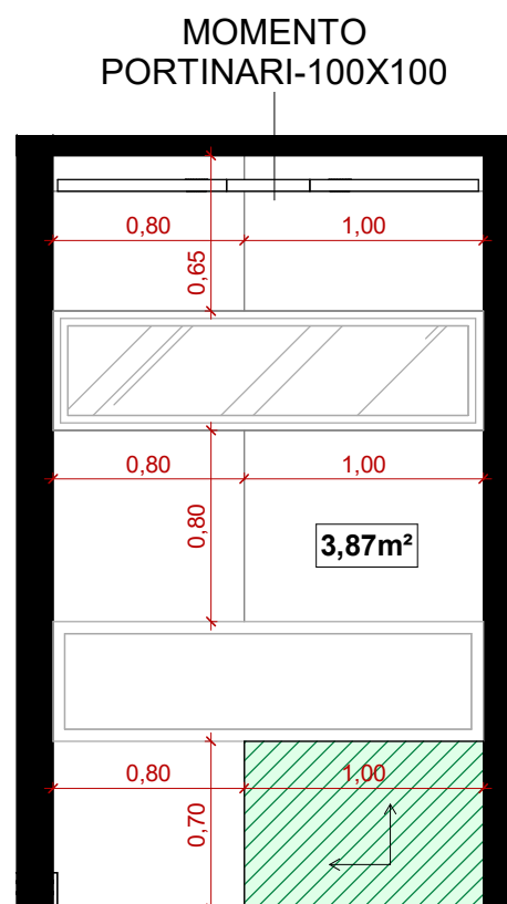
4 WC 02 - ELEVAÇÃO ESQUERDA 1 : 35
