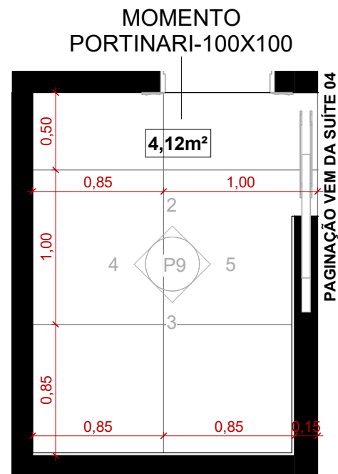
1 CLOSET 04 - PLANTA 1 : 35
