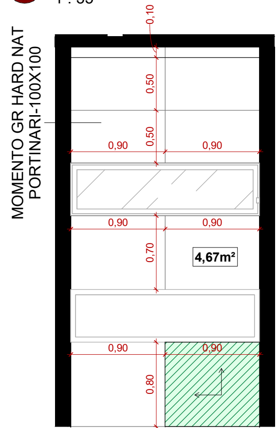
5 WC 01 - ELEVÇÃO LAT. DIREITA 1 : 35
