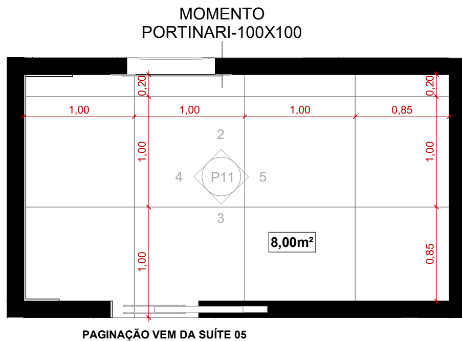
1 CLOSET 05 - PLANTA 1 : 35
