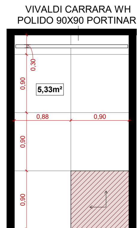
5 WC 10 - ELEVAÇÃO LAT. DIREITA 1 : 35
