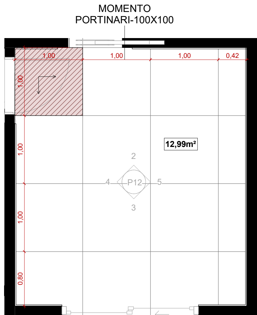
1 SUÍTE 05 - PLANTA 1 : 35
