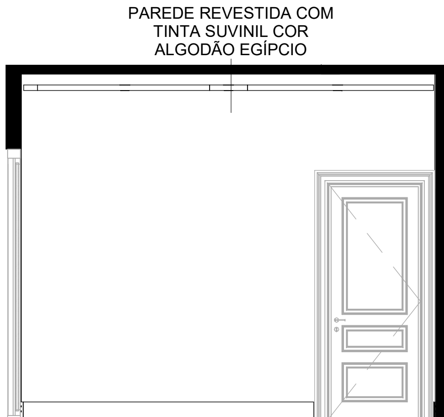
4 SUÍTE 05 - ELEVAÇÃO ESQUERDA 1 : 35
