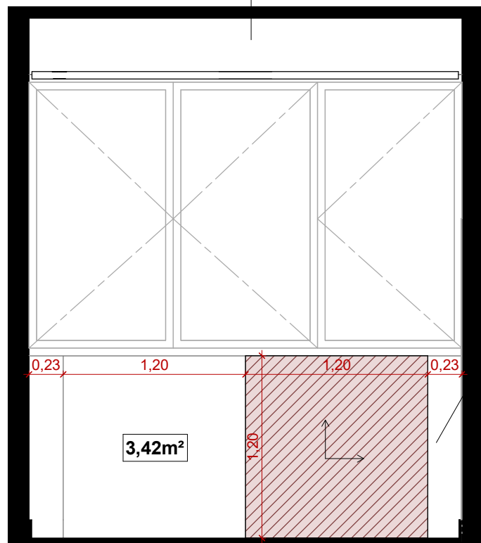
2 COZINHA (SALÃO) - ELEVAÇÃO FRONTAL 1 : 35
