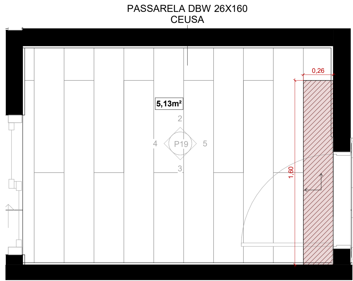
1 HOME OFFICE 01 - PAGINAÇÃO 1 : 20
