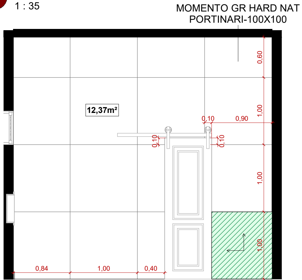
3 WC 01 - ELEVÇÃO POSTERIOR 1 : 35
