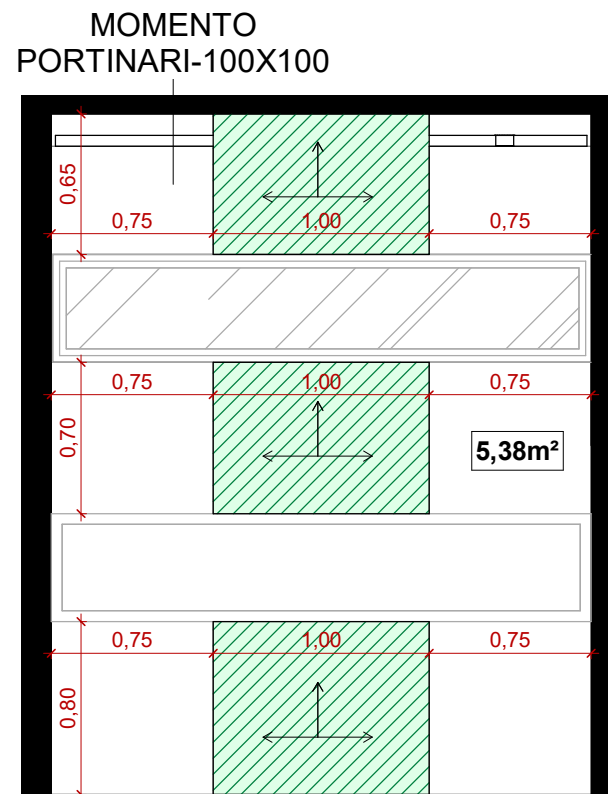
2 WC 04 - ELEVAÇÃO FRONTAL 1 : 35
