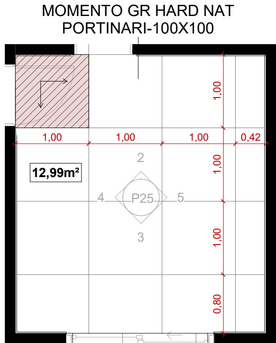
1 SUÍTE 01 - PAGINAÇÃO 1 : 50
