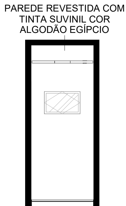
4 LAVABO - ELEVAÇÃO LAT. ESQUERDA 1 : 50
