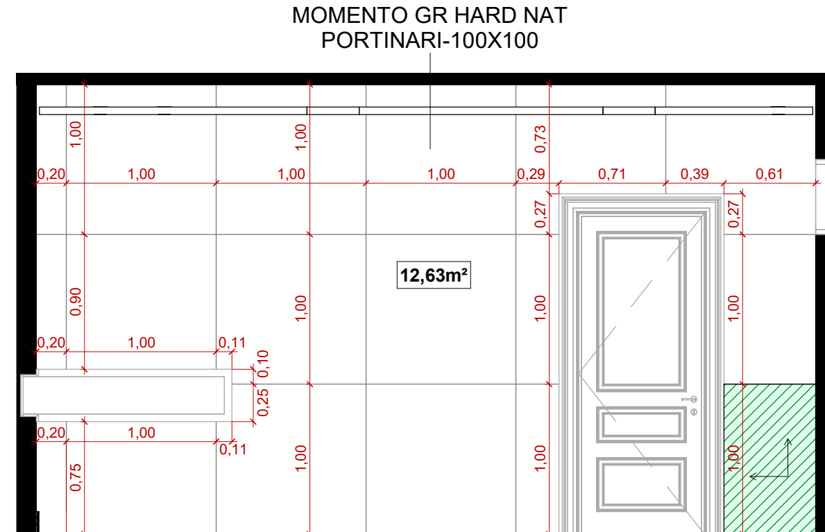
4 WC 06 - ELEVAÇÃO LAT. ESQUERDA 1 : 35
