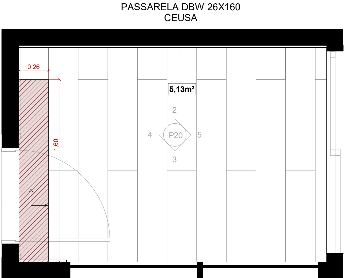
1 HOME OFFICE 02 - PAGINAÇÃO 1 : 20
