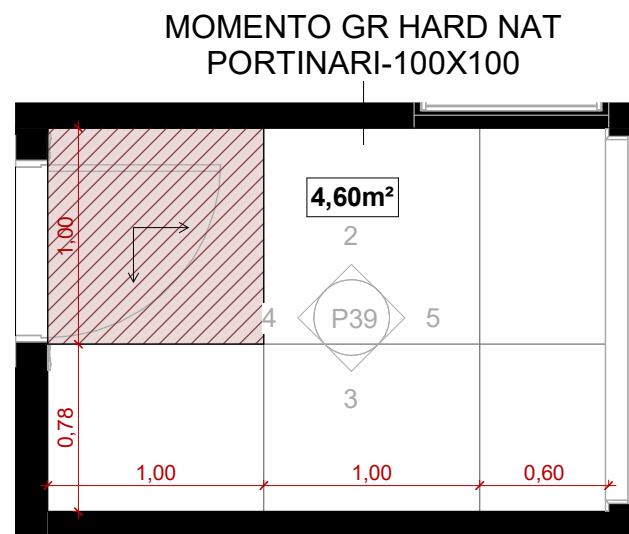
1 WC 07 - PAGINAÇÃO 1 : 35
