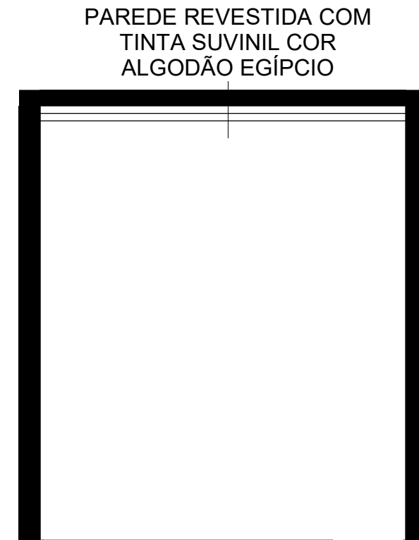
5 DEPÓSITO - BAR - ELEVAÇÃO LAT. DIREITA 1 : 35
