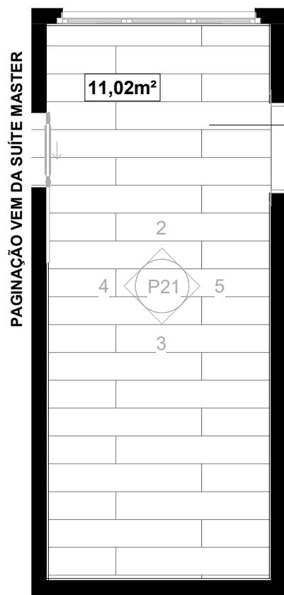
1 CLOSET 06 - PAGINAÇÃO 1 : 50
