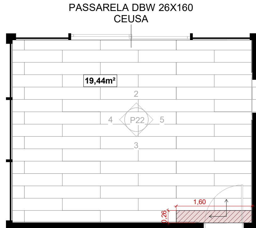
1 SUÍTE MASTER - PAGINAÇÃO 1 : 50
