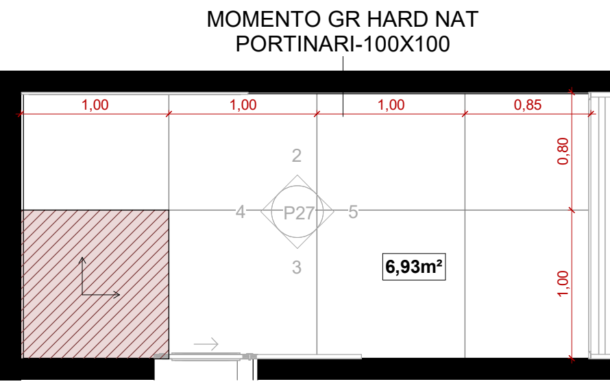
1 WC 01 - PAGINAÇÃO 1 : 35
