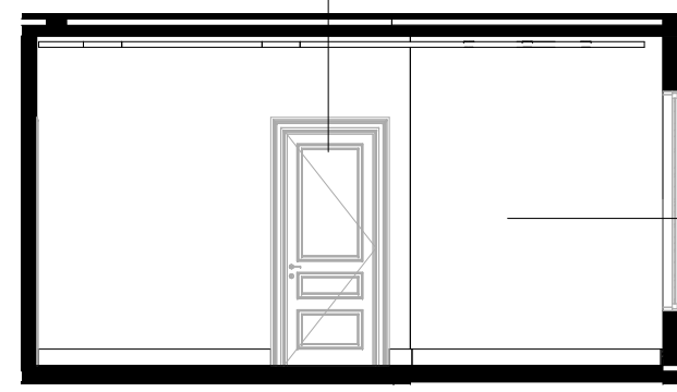
5 CIRCULAÇÃO - SUÍTE MASTER - ELEVação LAT. ESQUERDA 1 : 75
