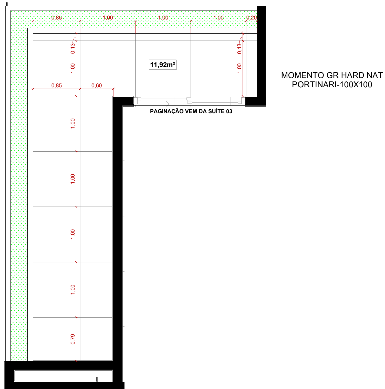
1 SUÍTE 03 - SACADA PLANTA 1 : 35
