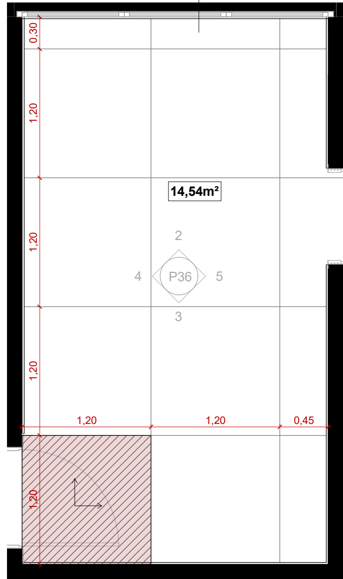
1 COZINHA (SALÃO) - PAGINAÇÃO 1 : 35
