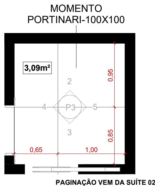
1 CLOSET 02 - PLANTA 1 : 35
