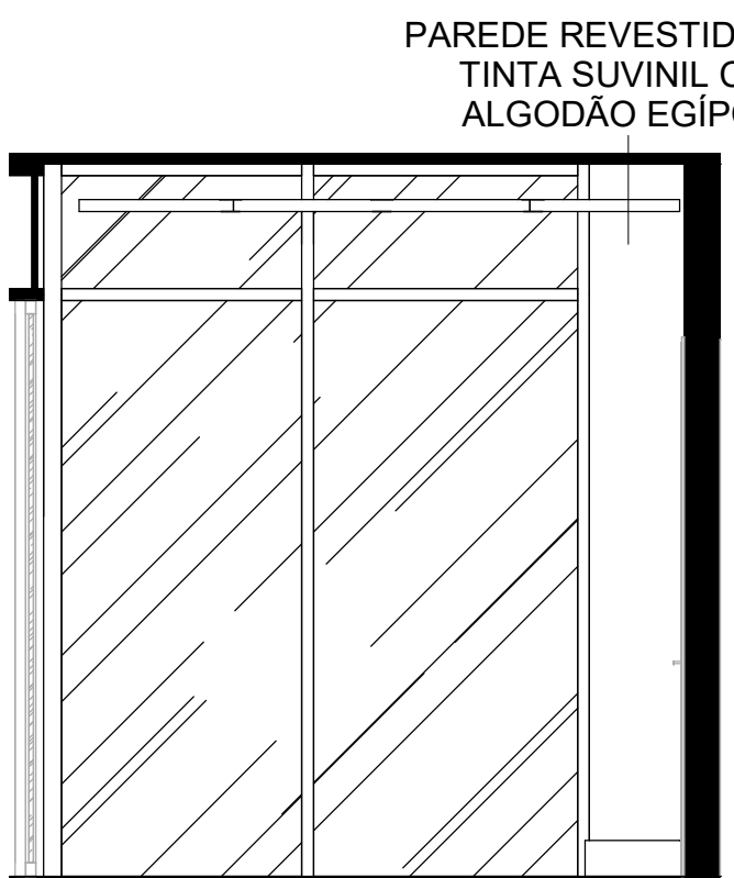
3 HOME OFFICE 02 - ELEVAÇÃO POSTERIOR 1 : 35
