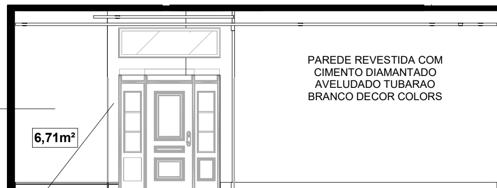
5 ESTAR/JANTAR - ELEVAÇÃO POSTERIOR
