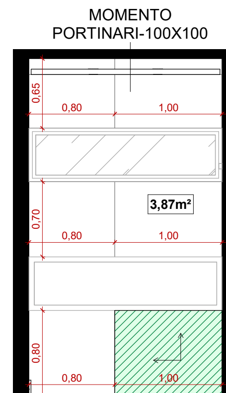
5 WC 05 - ELEVAÇÃO LAT. DIREITA 1 : 35
