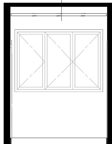
2 CLOSET 06 - ELEVAÇÃO FRONTAL 1 : 50
