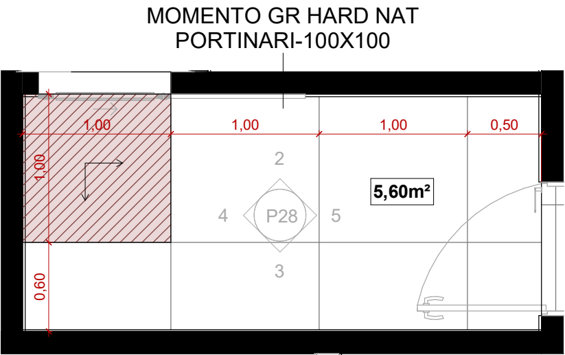
1 LAVANDERIA - PAGINAÇÃO 1 : 35
