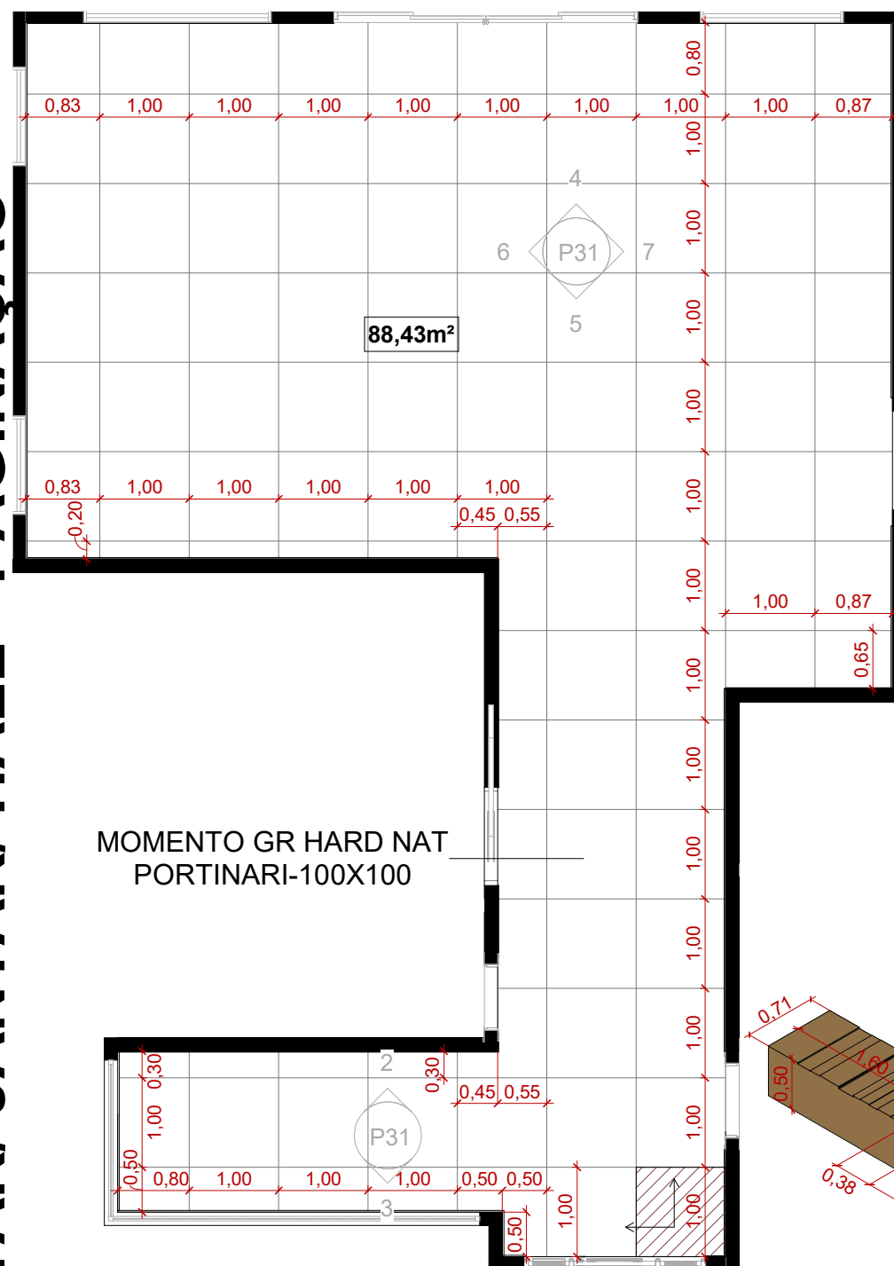
1 ESTAR/JANTAR/HALL - PAGINAÇÃO 1 : 75
