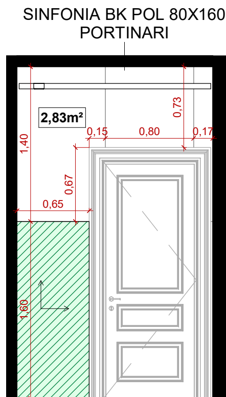
4 WC 09 - ELEVAÇÃO LAT. ESQUERDA 1 : 35
