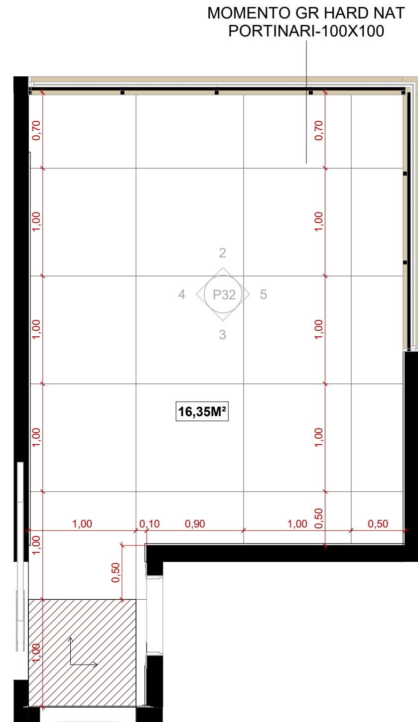
1 COZINHA (CASA) - PAGINAÇÃO 1 : 35
