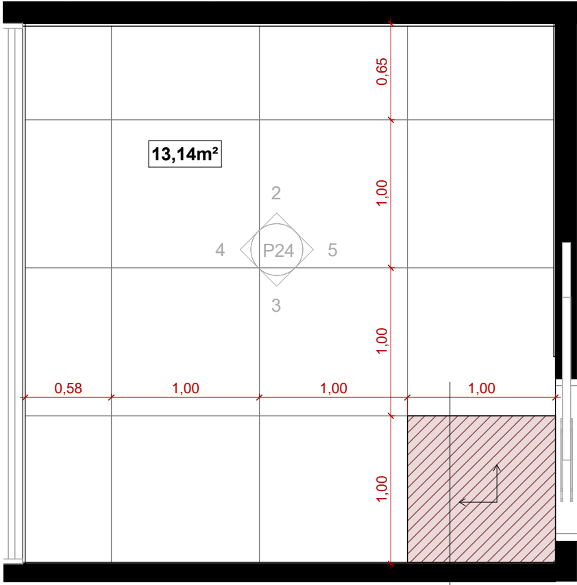
1 HOME THEATER - PAGINAÇÃO 1 : 35 MOMENTO GR HARD NAT PORTINARI-100X100
