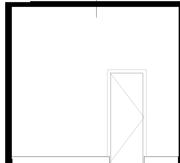
3 CLOSET 01 - ELEVAÇÃO POSTERIOR 1 : 50
