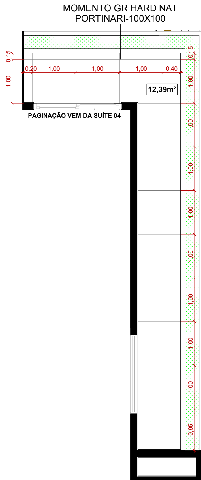
1 SUÍTE 04 - SACADA - PLANTA 1 : 50
