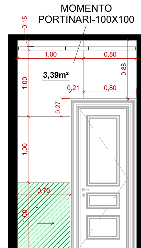
5 WC 02 - ELEVAÇÃO DIREITA 1 : 35
