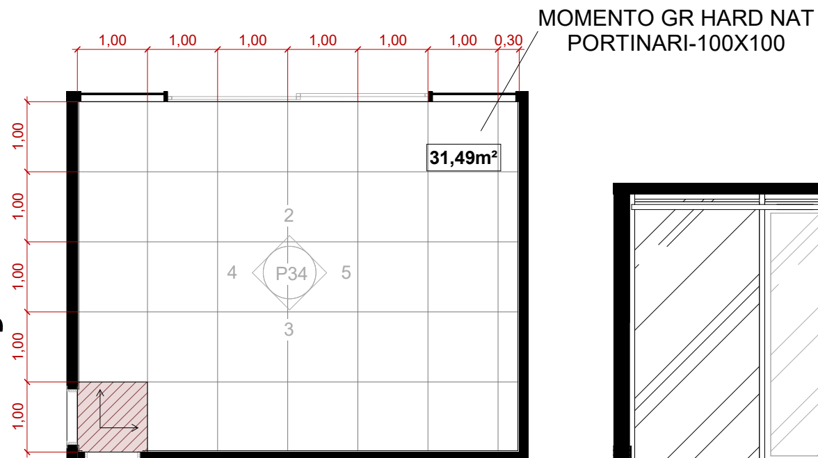
1 ACADEMIA - PAGINAÇÃO 1 : 75
