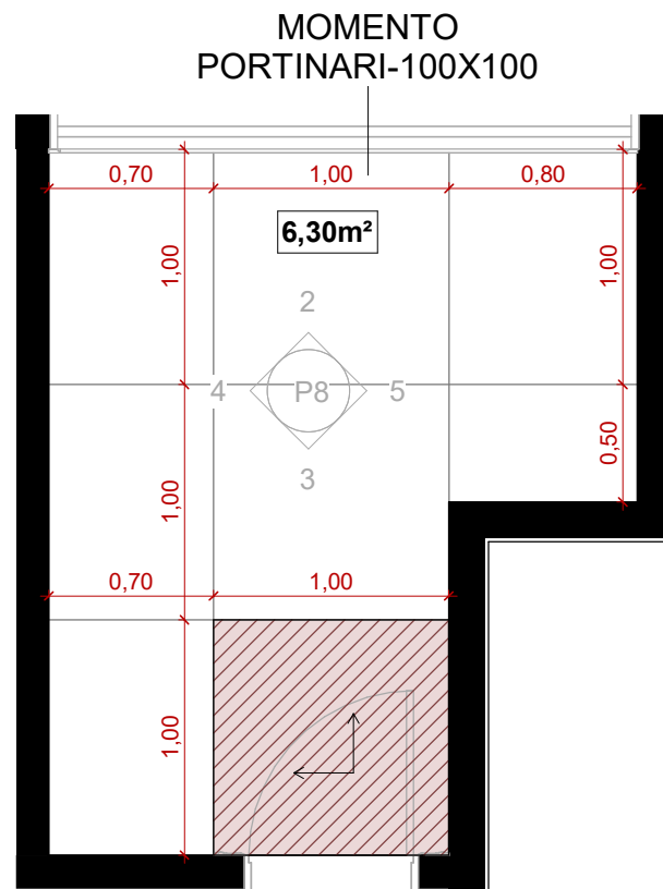
1 WC 04 - PLANTA 1 : 35
