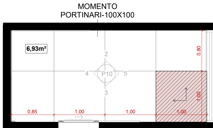
1 WC 05 - PLANTA 1 : 35
