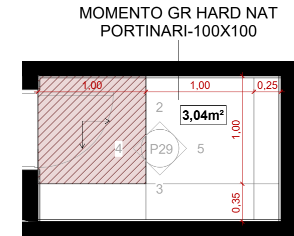
1 DESPENSA - PAGINAÇÃO 1 : 35
