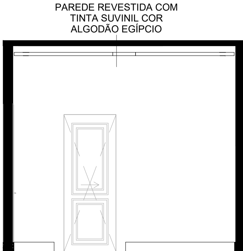
2 SUÍTE 05 - ELEVAÇÃO FRONTAL 1 : 35
