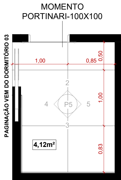
1 CLOSET 03 - PLANTA 1 : 35
