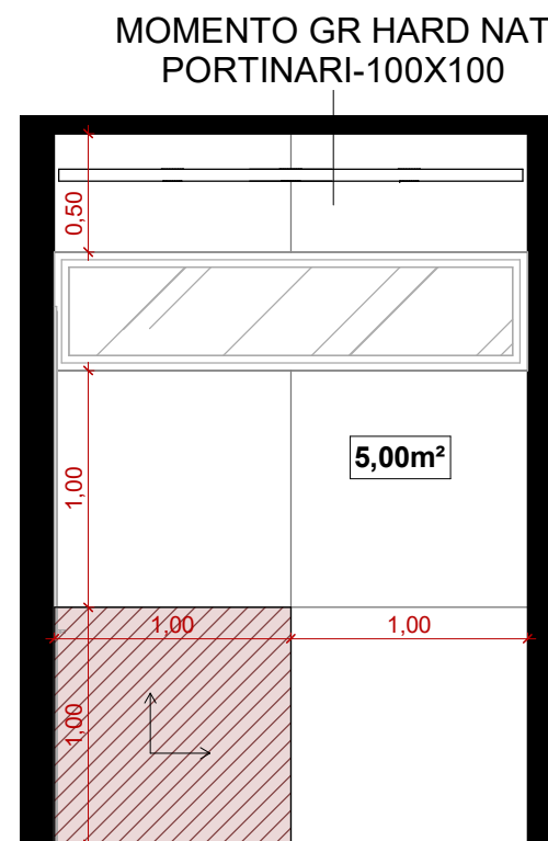
2 WC 06 - ELEVAÇÃO FRONTAL 1 : 35
