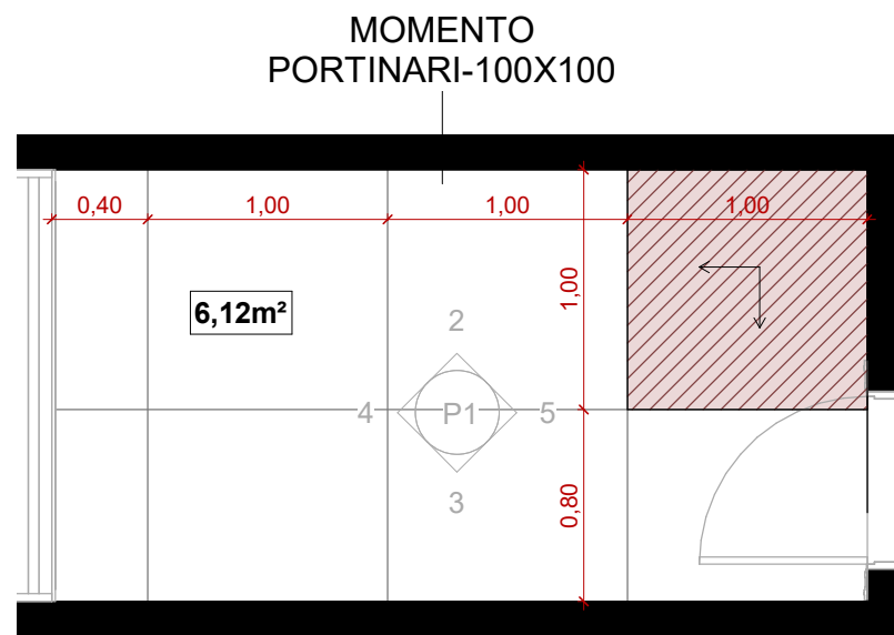
1 WC 02 - PLANTA 1 : 35
