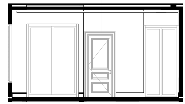
4 CIRCULAÇÃO - SUÍTE MASTER - ELEVação LAT. DIREITA 1 : 75
