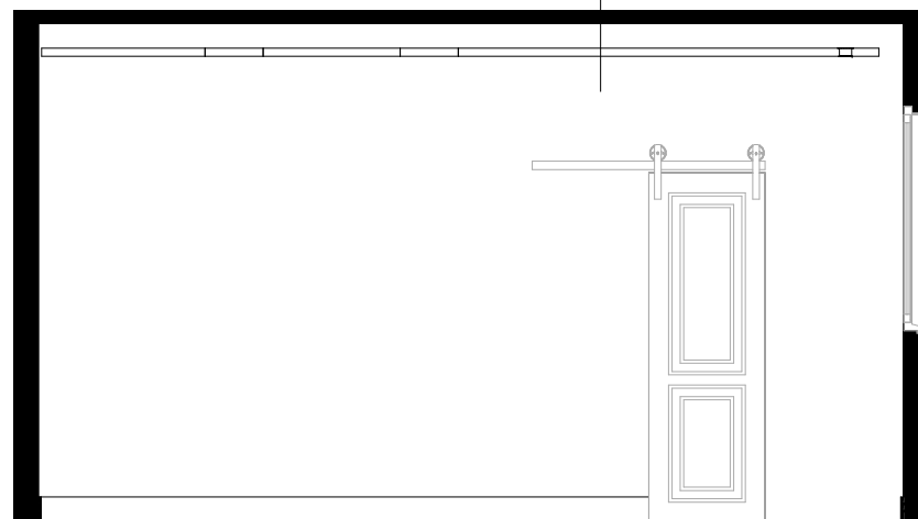
4 CLOSET 06 - ELEVAÇÃO LAT. ESQUERDA 1 : 50
