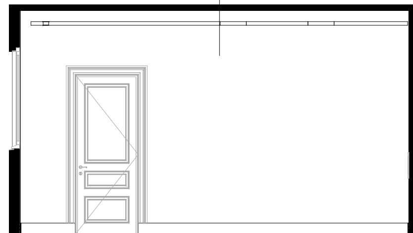
5 CLOSET 06 - ELEVAÇÃO LAT. DIREITA 1 : 50
