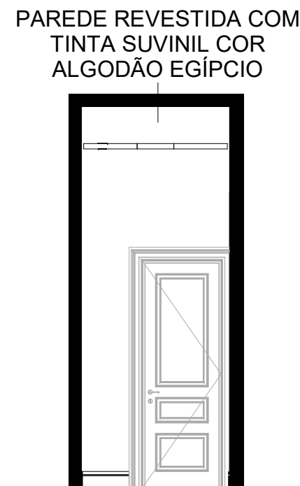
5 LAVABO - ELEVAÇÃO LAT. DIREITA 1 : 50
