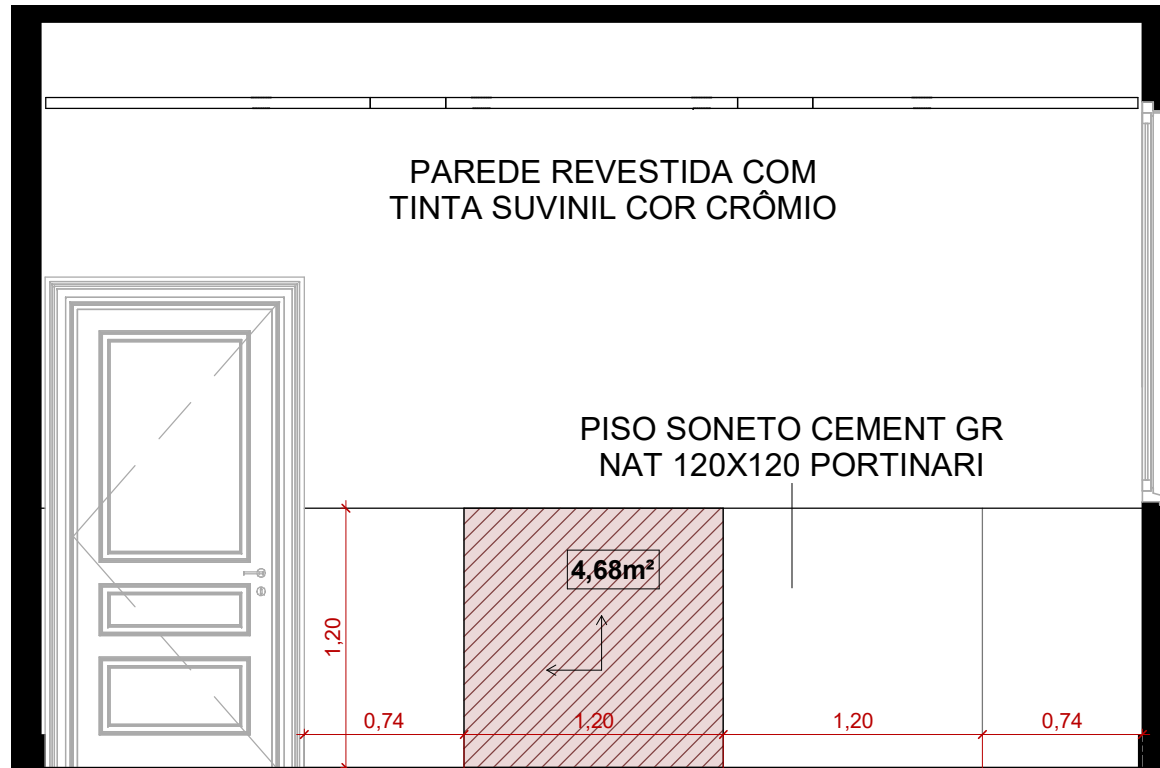
4 COZINHA (SALÃO) - ELEVAÇÃO LAT. ESQUERDA 1 : 35
