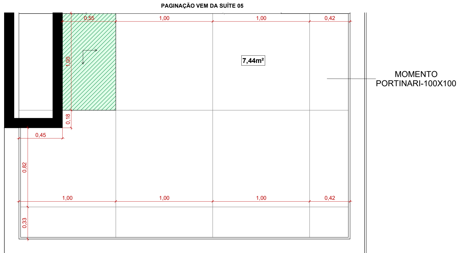
1 SUÍTE 05 - SACADA PLANTA 1 : 20
