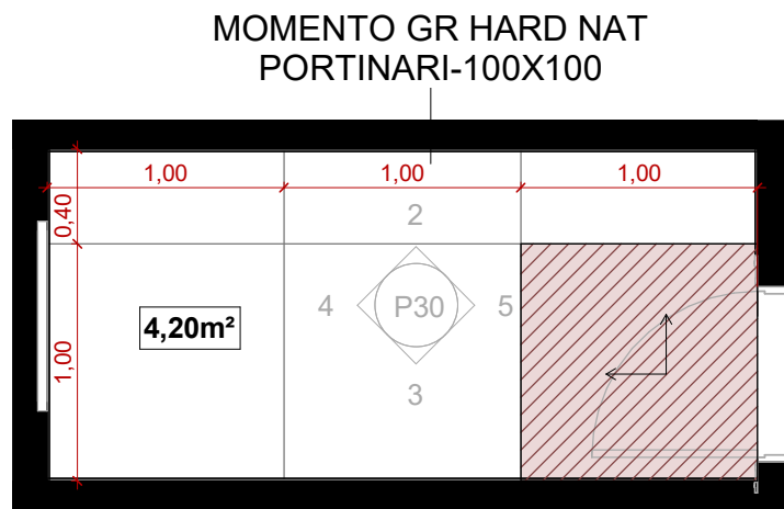
1 LAVABO - PAGINAÇÃO 1 : 35
