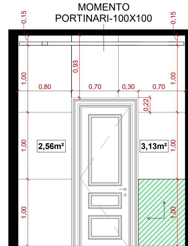
3 WC 04 - ELEVAÇÃO POSTERIOR 1 : 35
