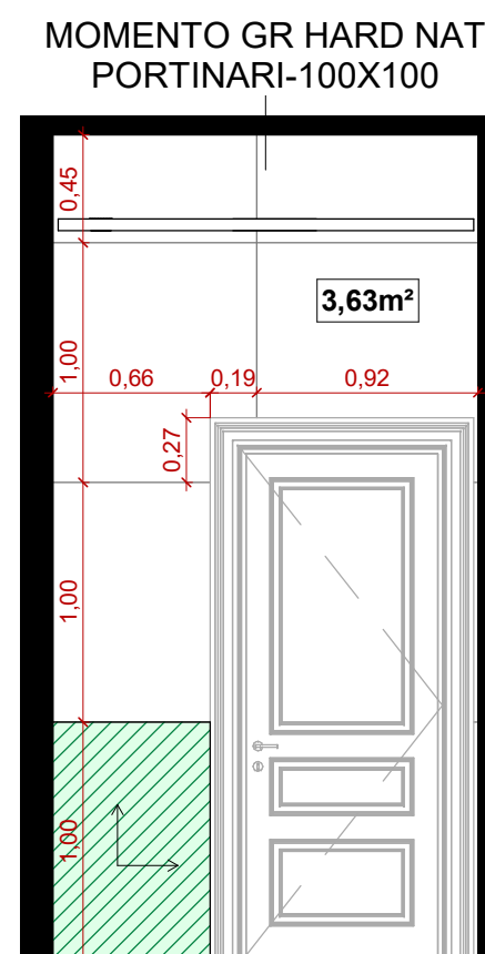
4 WC 07 - ELEVAÇÃO LAT. ESQUERDA 1 : 35
