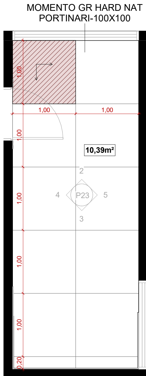
1 WC 06 - PAGINAÇÃO 1 : 35
